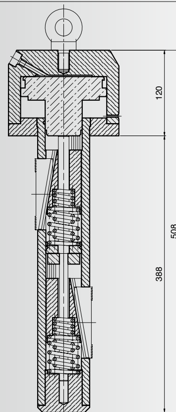
SOLLEVATORE PNEUMO - MECCANICO 3" BOBBIN LIFTING HEADER 3"
