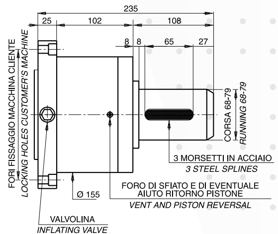
TESTATA PNEUMO - MECCANICA CON RITORNO A MOLLA ANIME Ø 152
